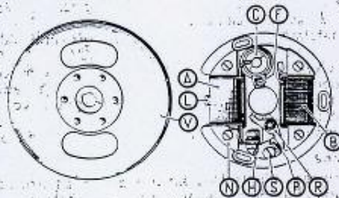
fig. 3 - Magnete alternatore volante
